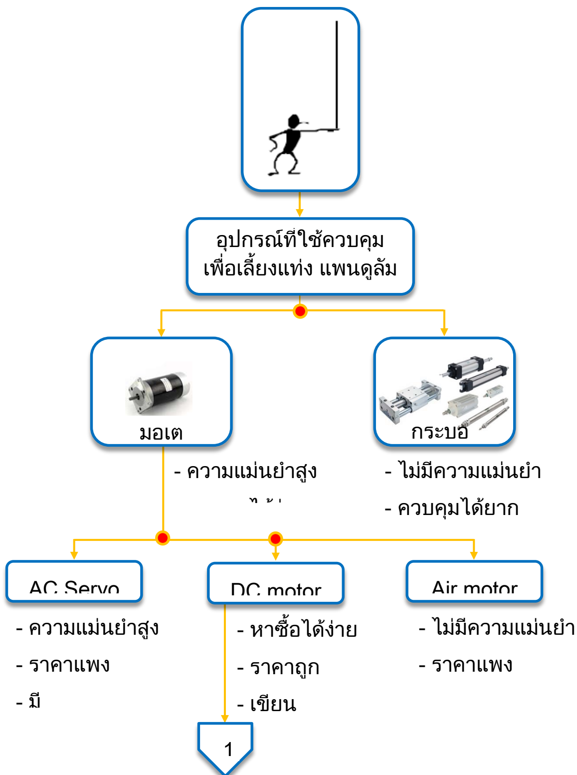
ภาพที่ ก-1 แนวคิดในการสร้างชุดควบคุมระบบแพนดูลัมผกผัน
