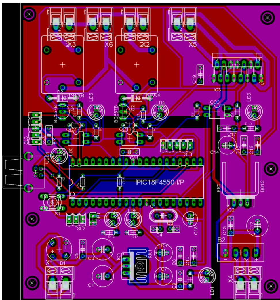
รูปที่ ก-1 ลายวงจรไฟฟ้าของไมโครคอนโทรลเลอร์และ ชุดขับ L298
