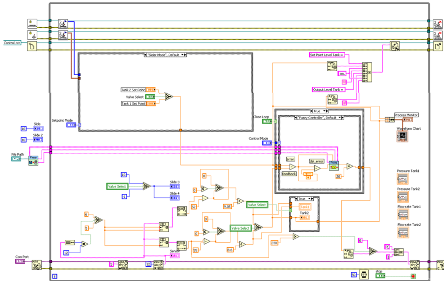
รูปที่ ค-1 หน้าต่างสำหรับการเขียนโปรแกรมการควบคุมระดับน้ำ
