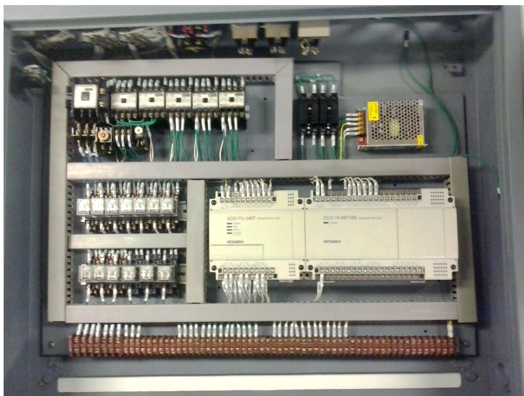
ภาพที่ ข-6 ติดตั้งอุปกรณ์ไฟฟ้าลงในตู้ควบคุม
