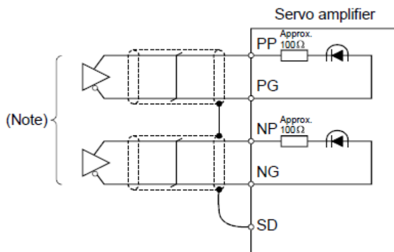
ภาพที่ ก-3 วงจรที่สั่งให้ AC Servo Motor หมุนและกำหนดทิศทางการหมุน
