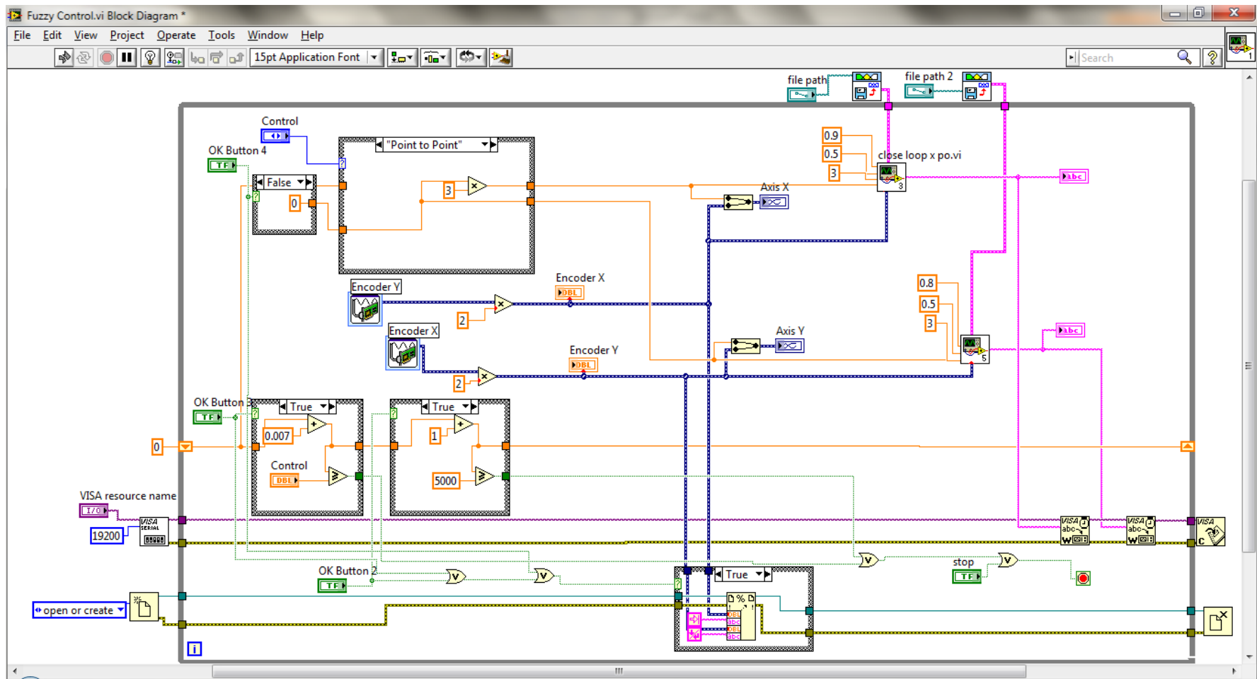
ภาพที่ ค-4 บล็อกไดอะแกรมการควบคุมแบบฟัซซี่
