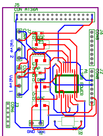
ภาพที่ ข-1 วงจรขับและควบคุมทิศทางวาล์ว (Drive and Direction)
