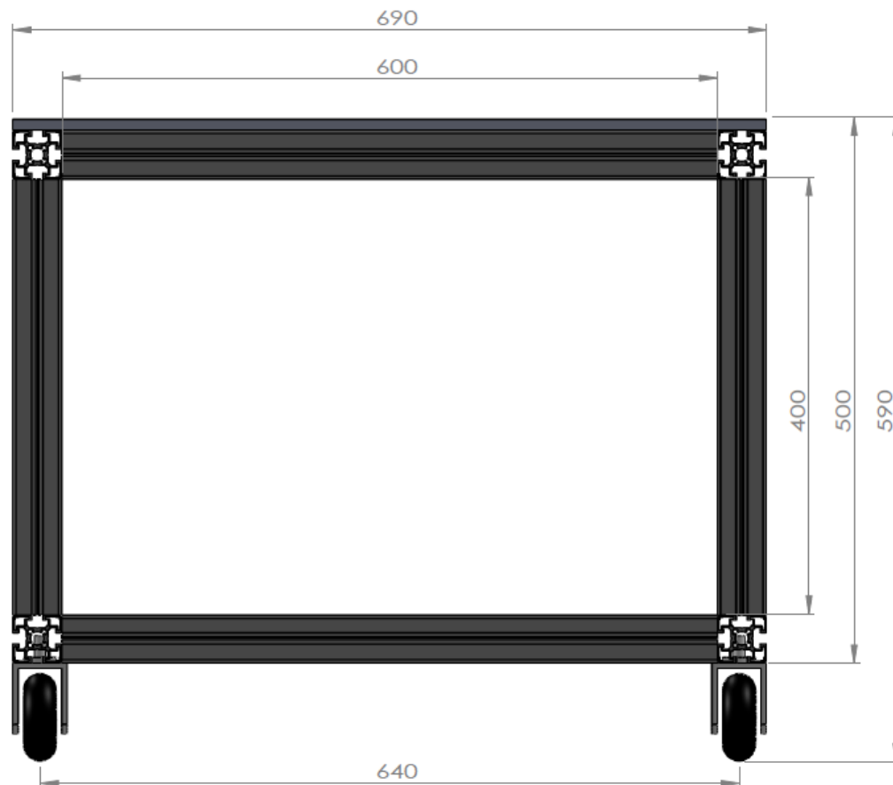
ภาพที่ ข-1 แบบโต๊ะถังรองถังน้ำมันไฮดรอลิกส์
