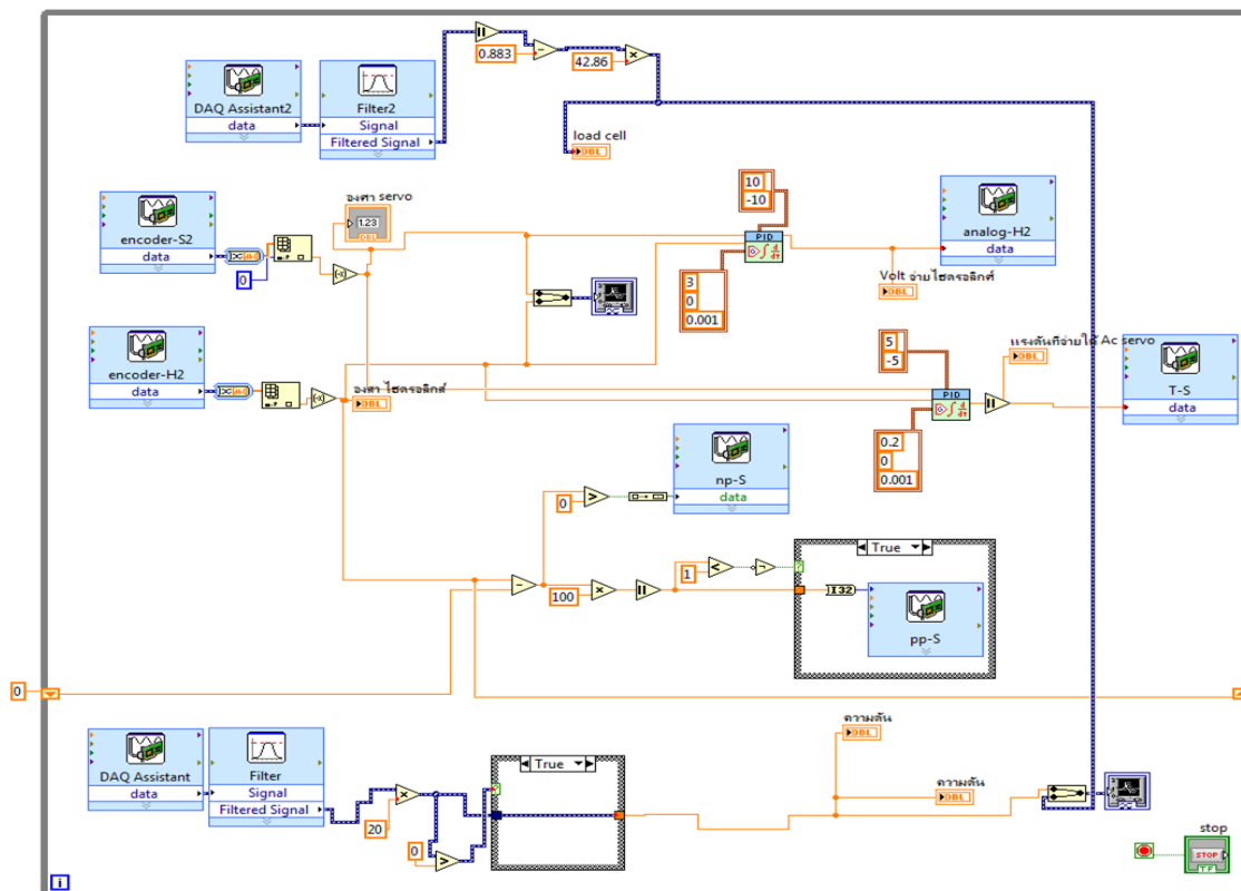
ภาพที่ ข-1 โปรแกรมที่ใช้ในการควบคุม แบบ P – P ไม่มีการชดเชยแรงเสียดทาน
