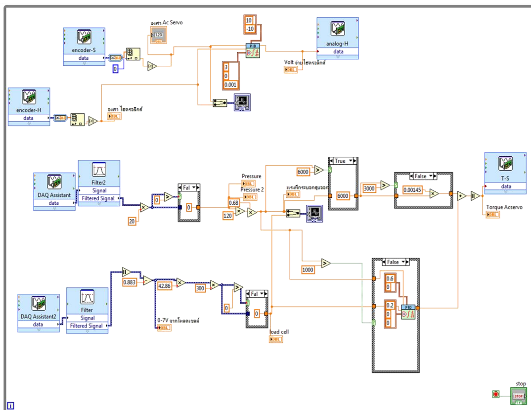
ภาพที่ ข-3 โปรแกรมที่ใช้ในการควบคุม แบบ P – F ไม่มีการชดเชยแรงเสียดทาน
