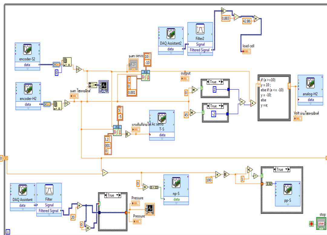
ภาพที่ ข-4 โปรแกรมที่ใช้ในการควบคุม แบบ P – F มีการชดเชยแรงเสียดทาน
