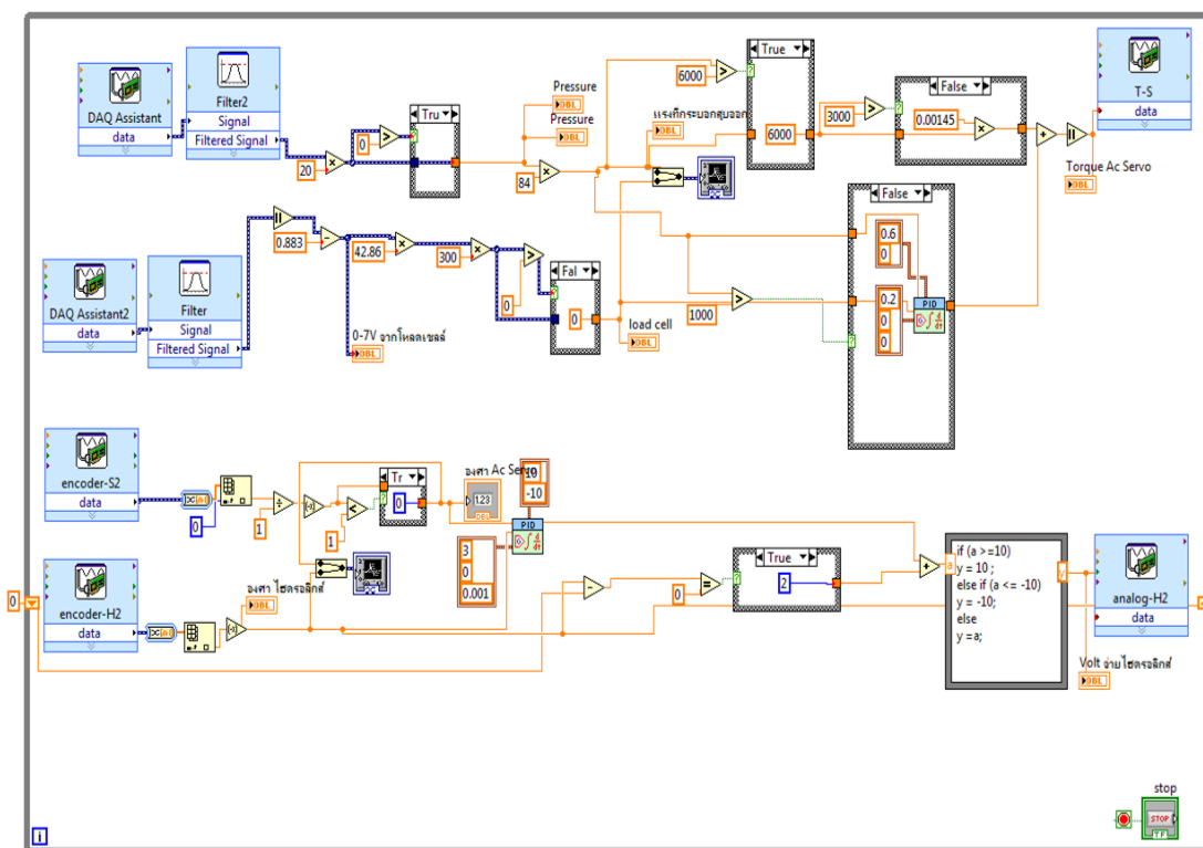
ภาพที่ ข-2 โปรแกรมที่ใช้ในการควบคุม แบบ P – P มีการชดเชยแรงเสียดทาน
