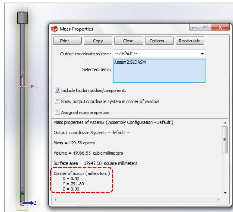
ภาพที่ ค-1 หาจุด CG ของแท่งของแท่งแปนดูลัมในโปรแกรม Solid Work
